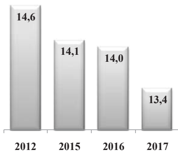
Смертность от всех причин на 1000 человек
