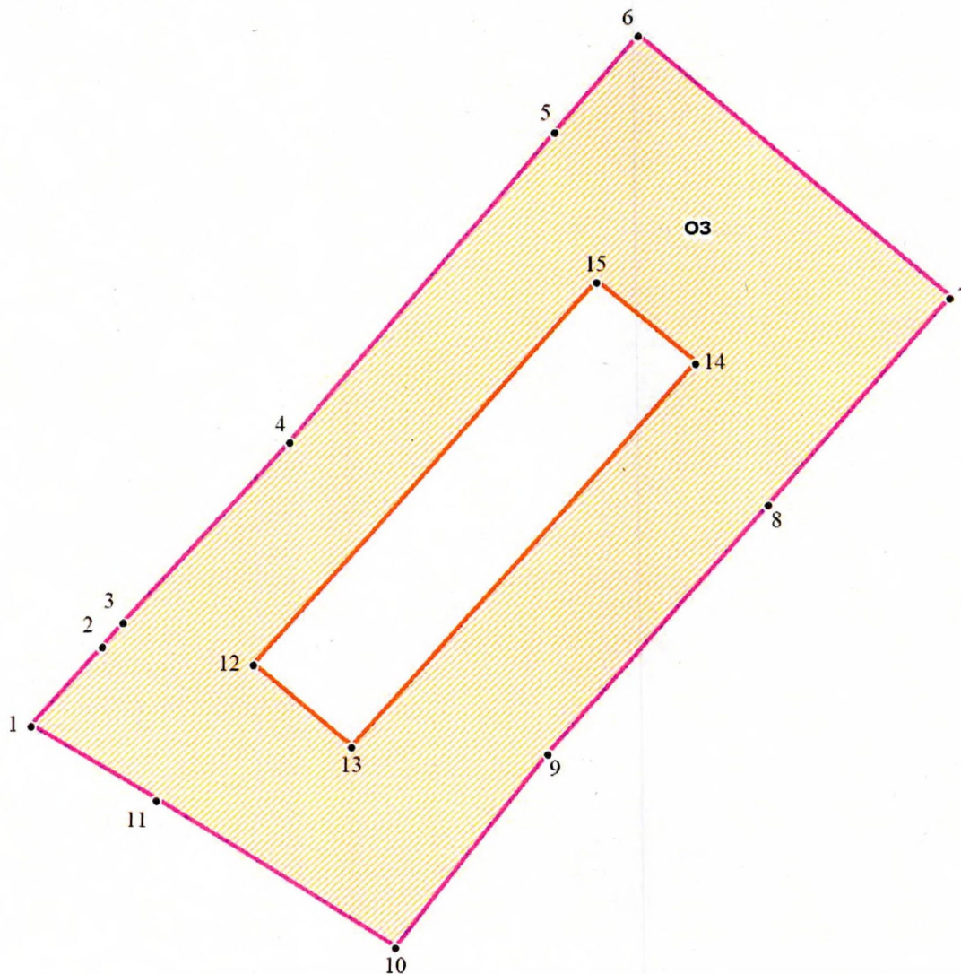
План характерных (поворотных) точек границ охранной зоны (ОЗ)
