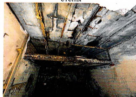
Подвал. Помещение в С-В исторической пристройке от 1934 г. Плоское перекрытие, кирпичные стены
